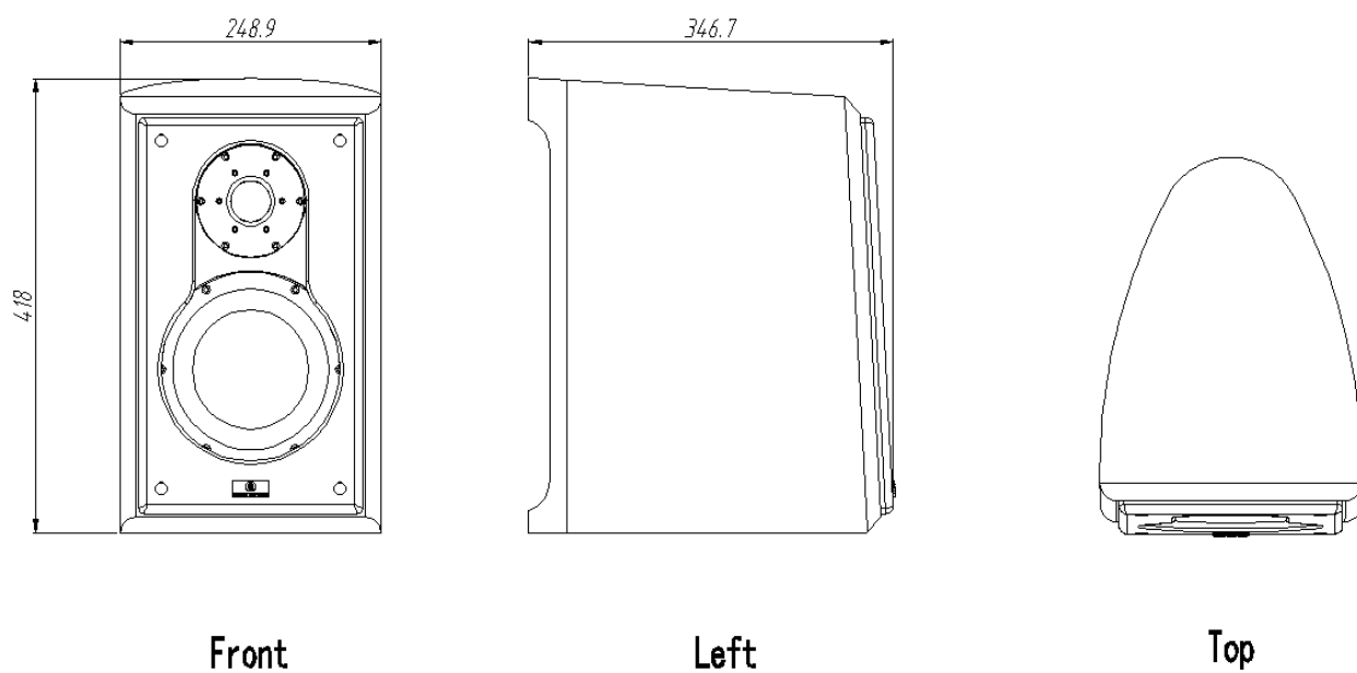
三视图
