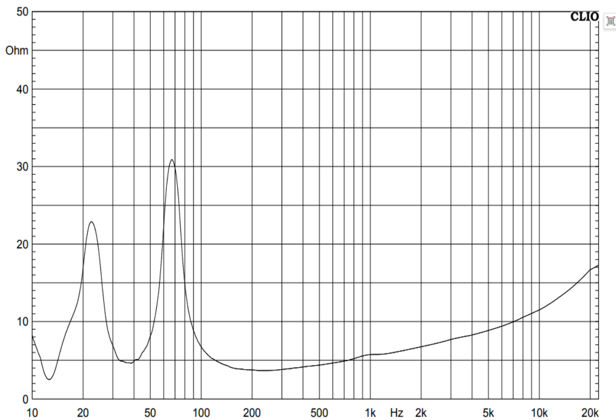
阻抗曲线
