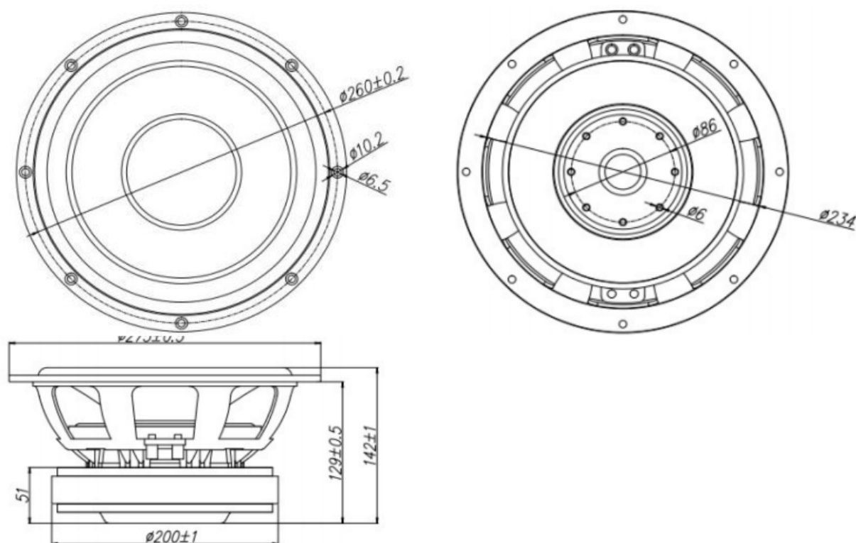
三视图
