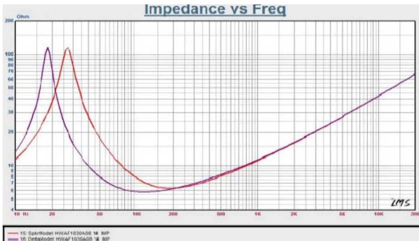
阻抗曲线
