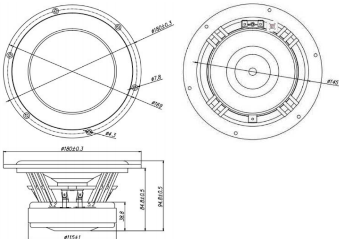
三视图
