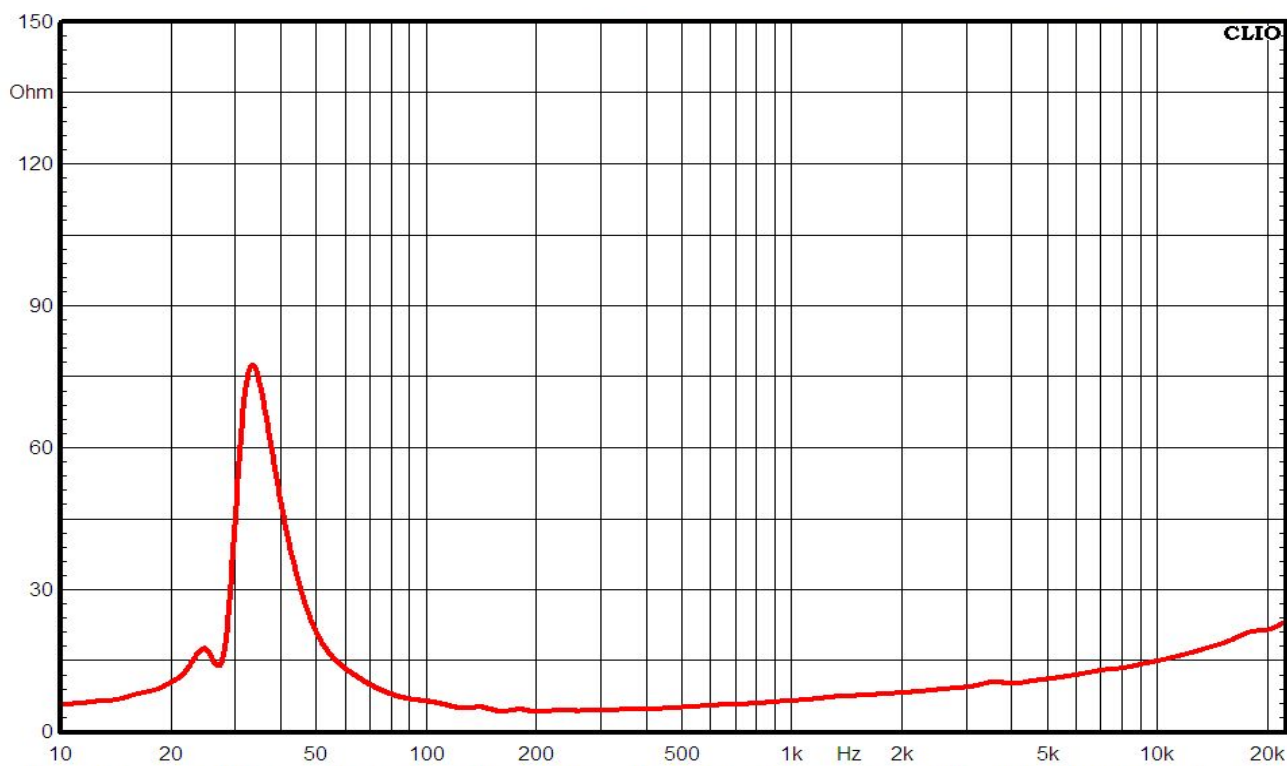
阻抗曲线
