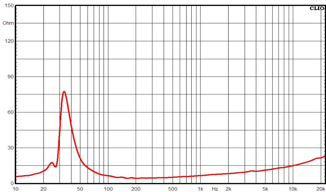
阻抗曲线
