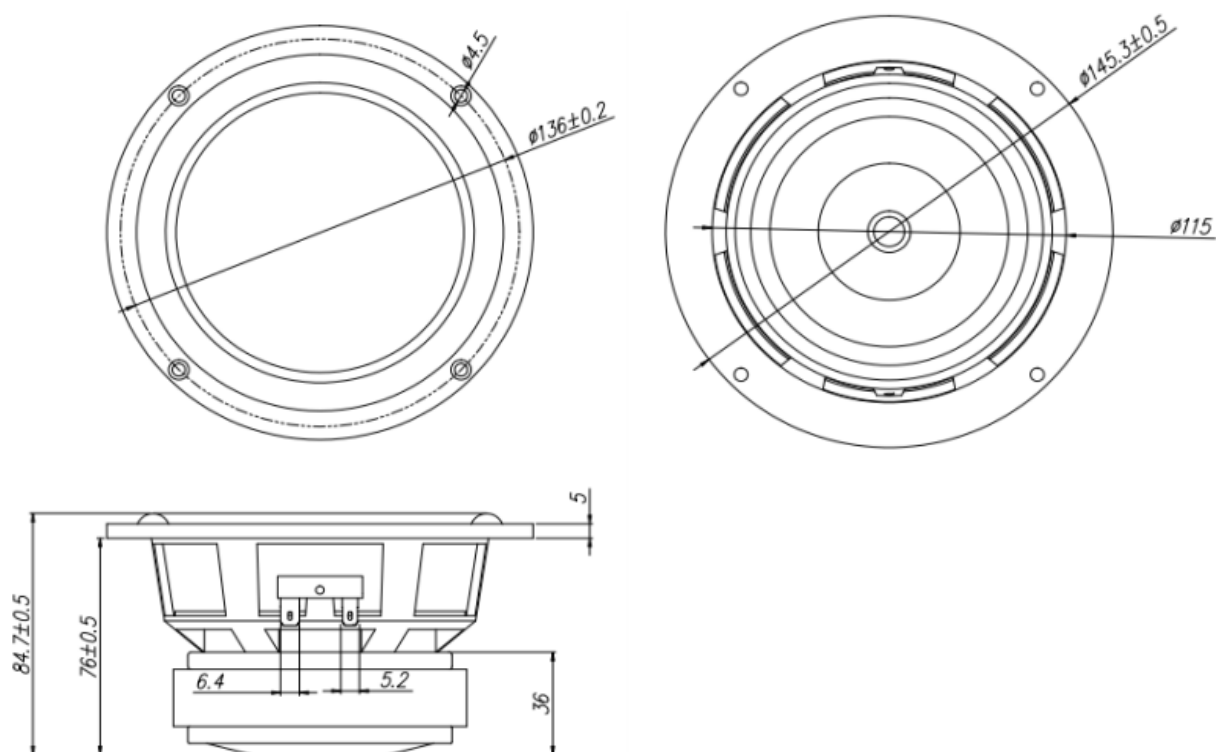
三视图
