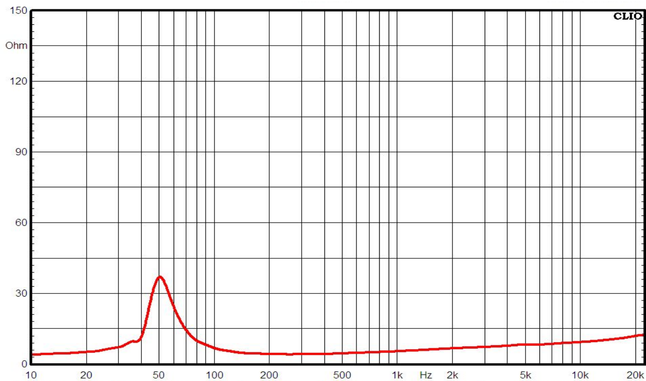
阻抗曲线
