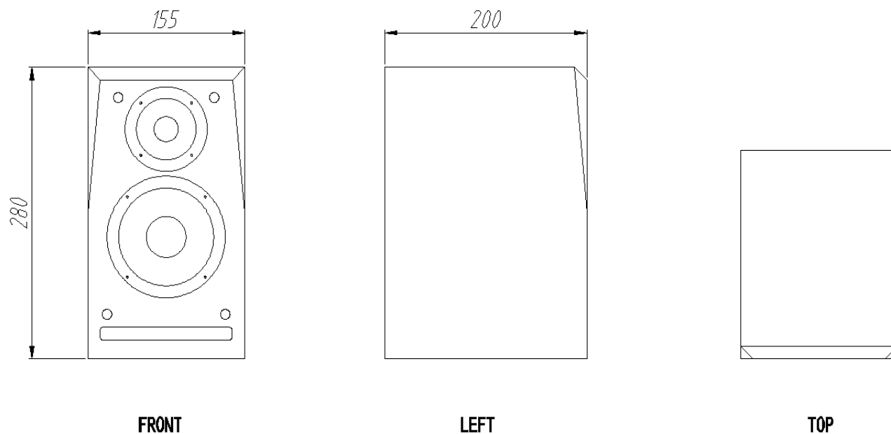
三视图
