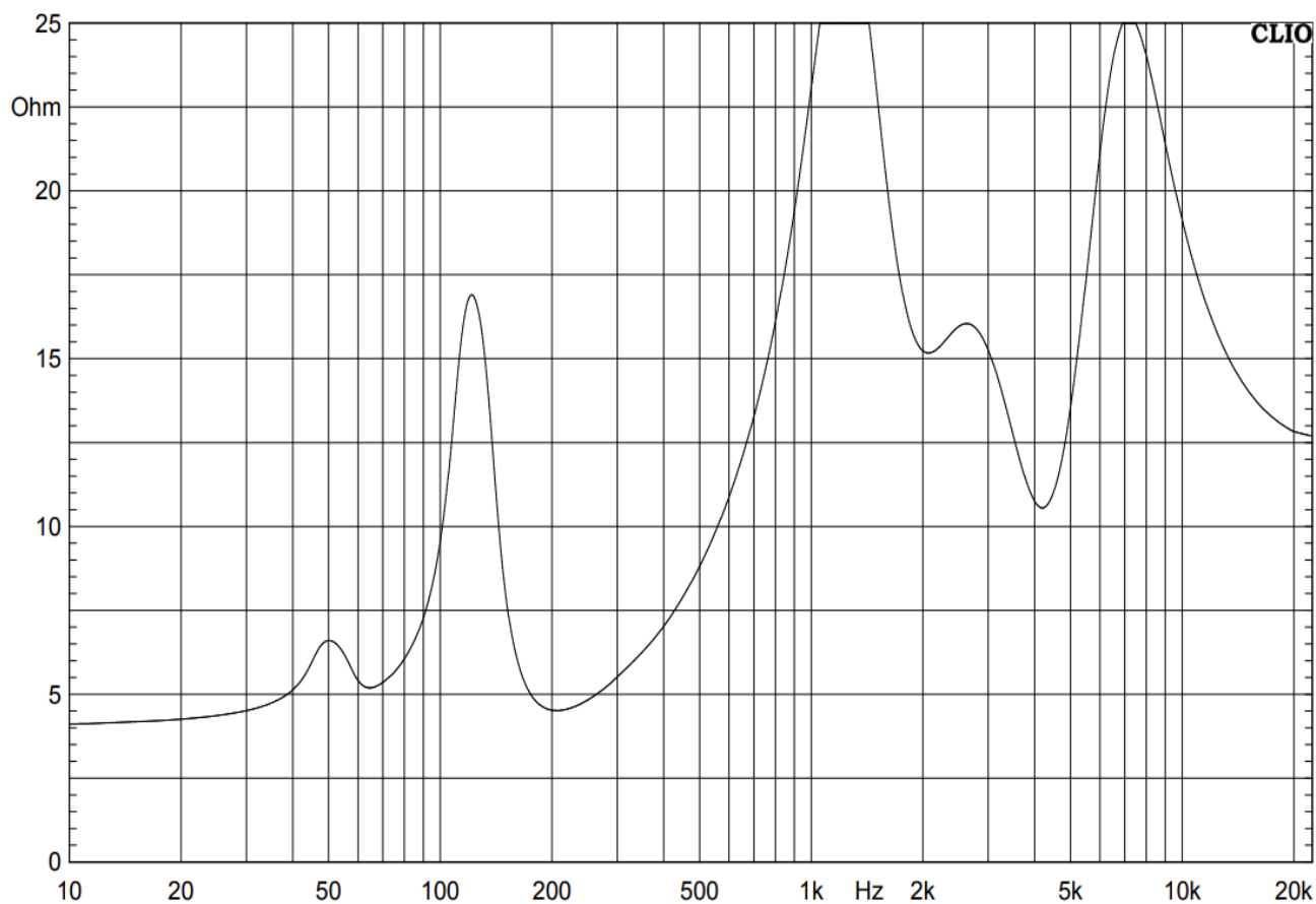
阻抗曲线
