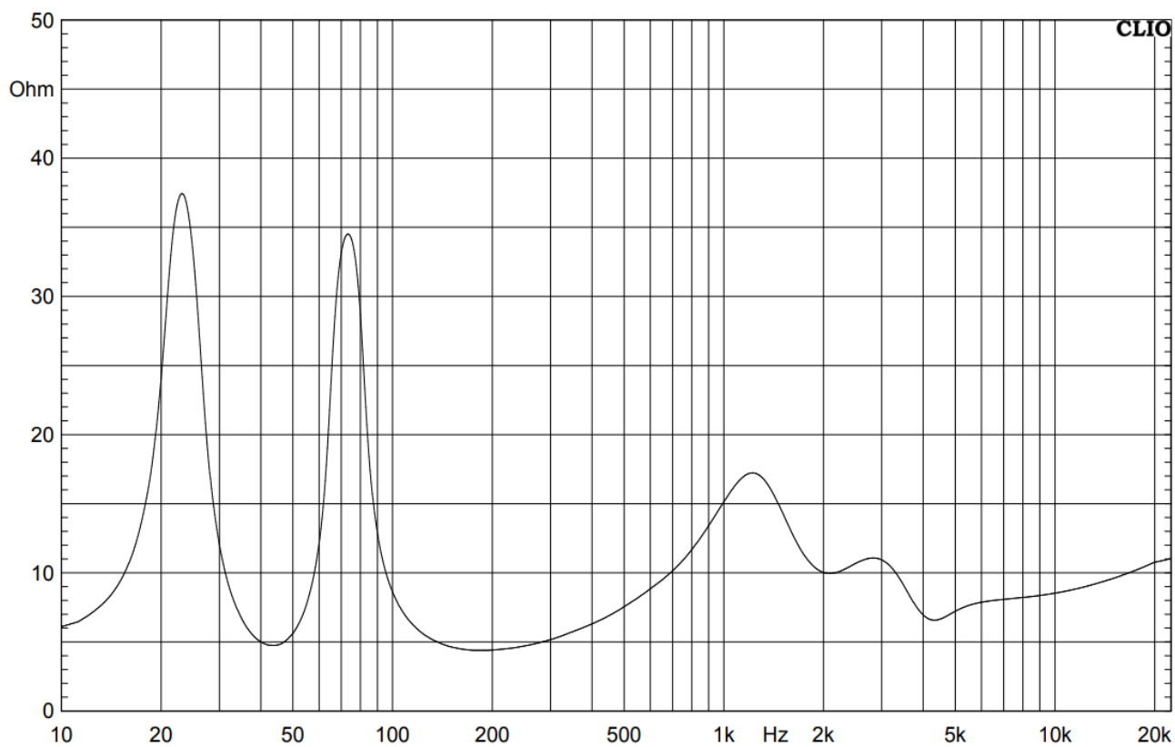
阻抗曲线
