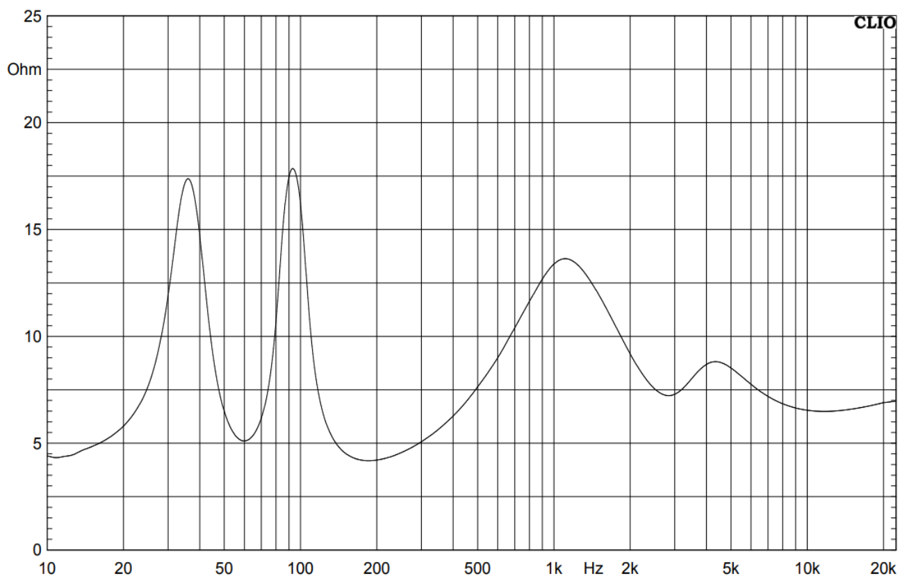
阻抗曲线
