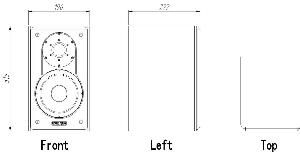
三视图
