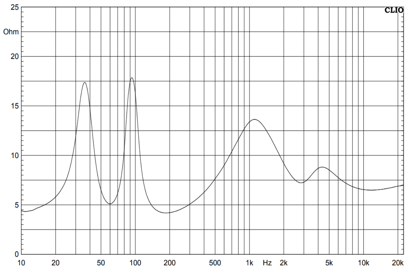
阻抗曲线
