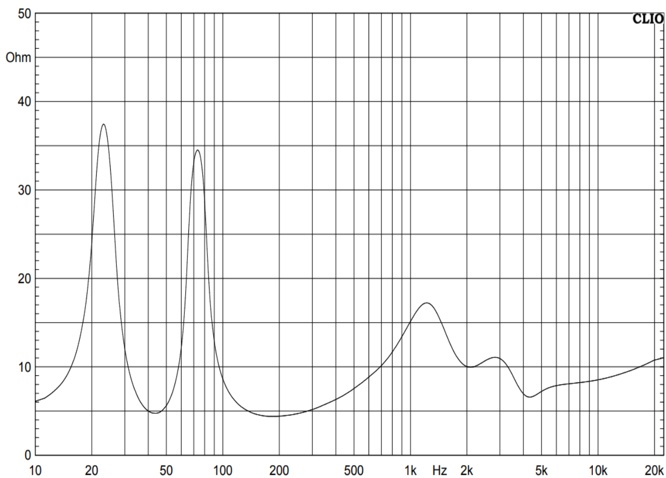
阻抗曲线
