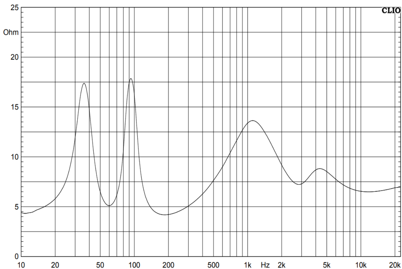
阻抗曲线
