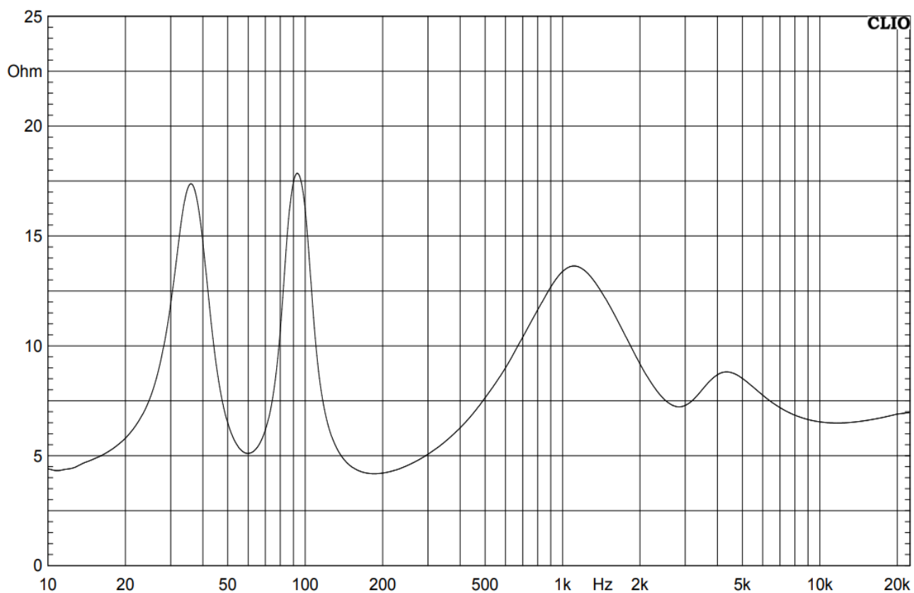
阻抗曲线
