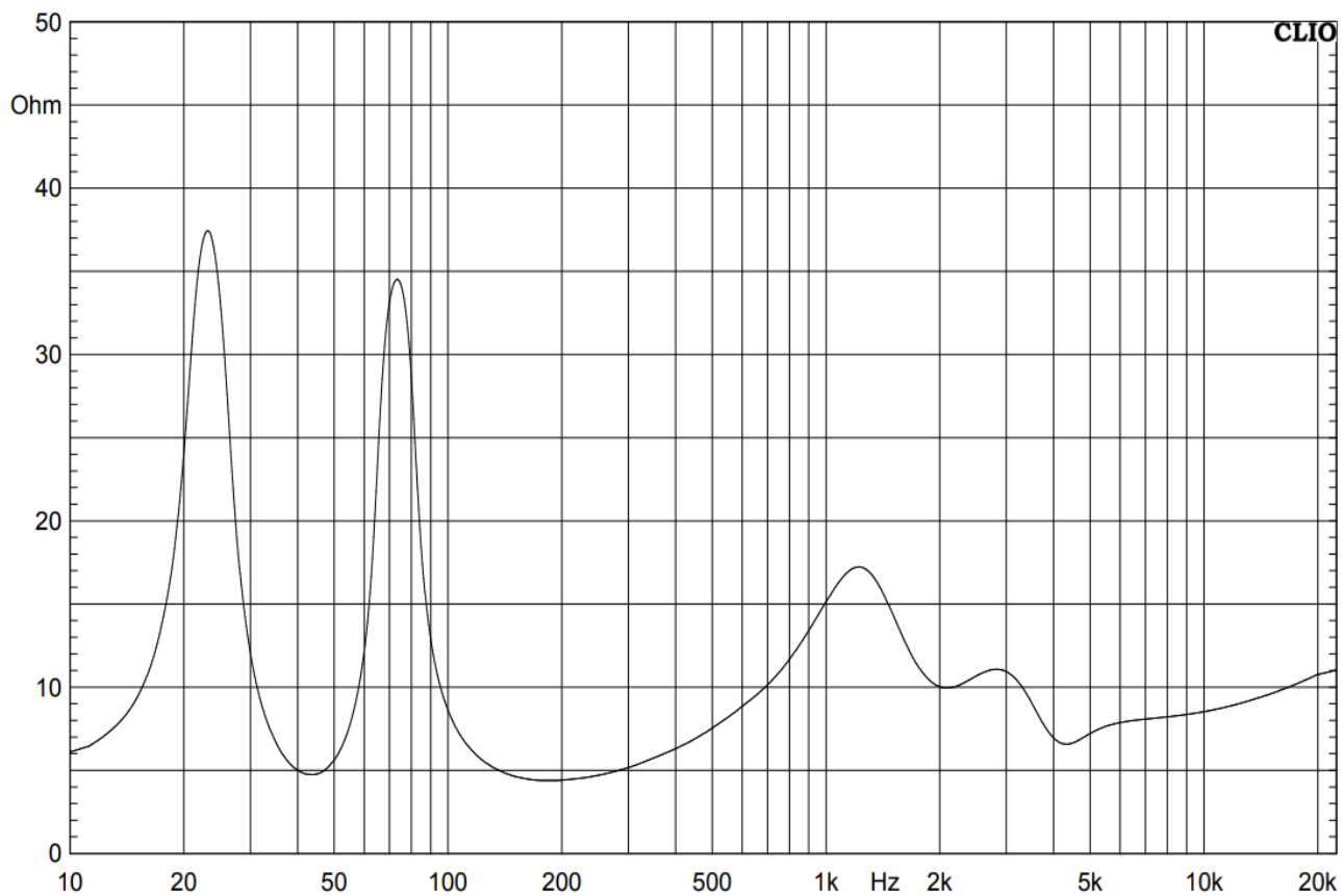
阻抗曲线
