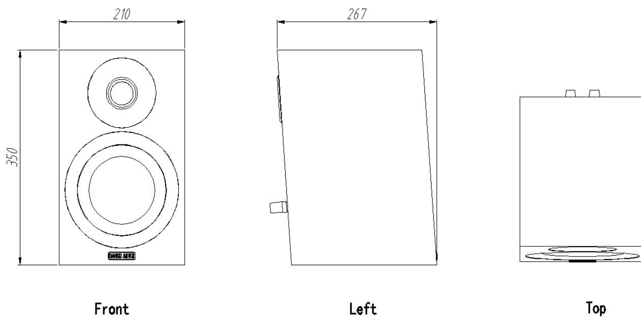
三视图
