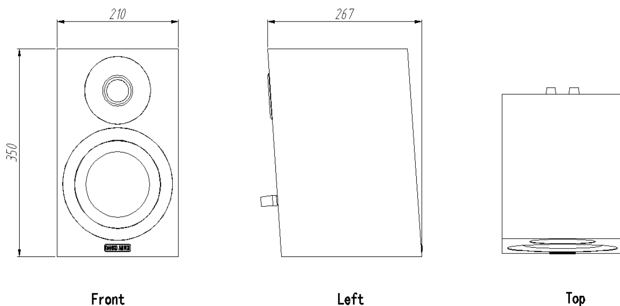
三视图
