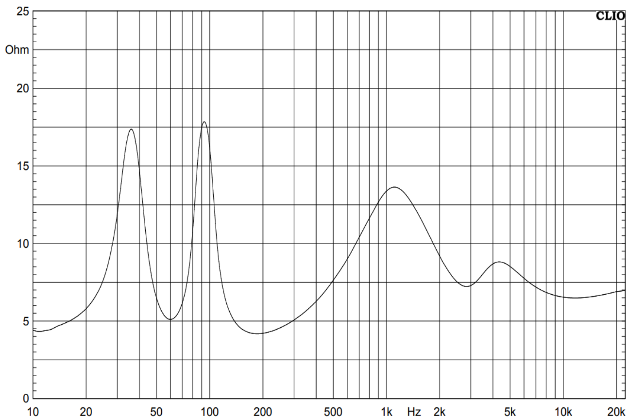
阻抗曲线
