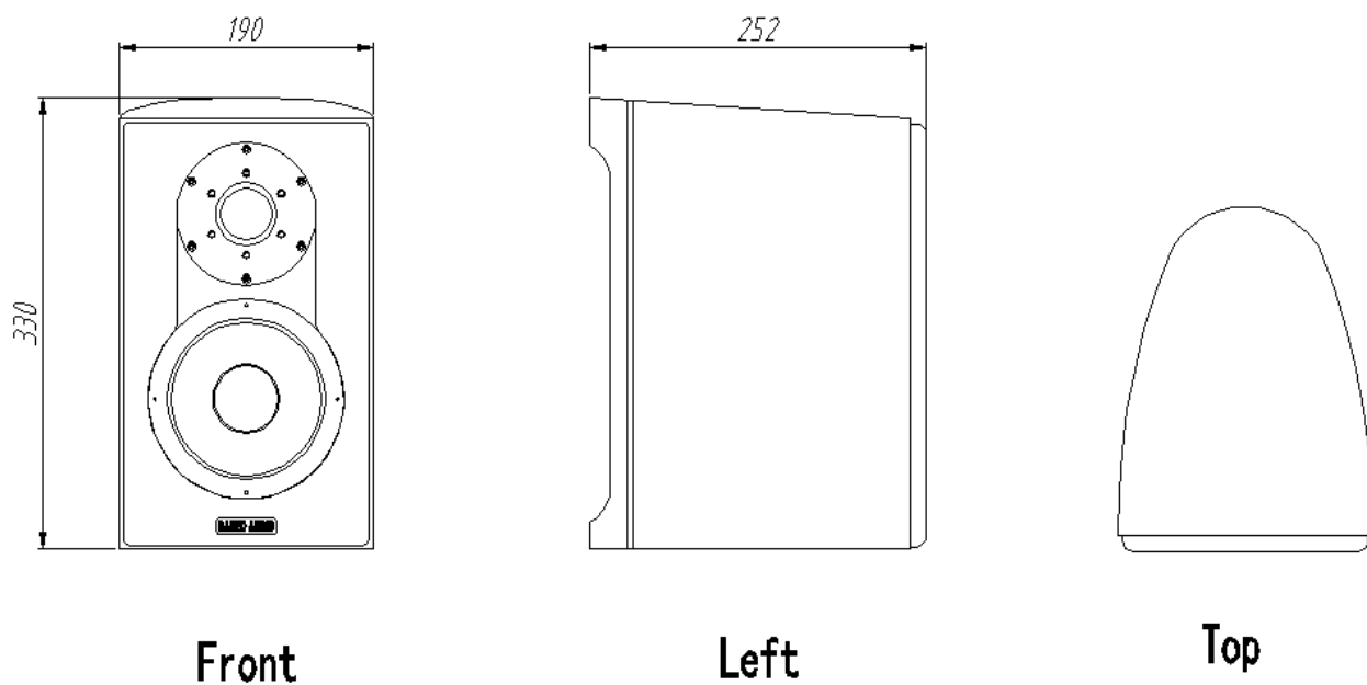
三视图
