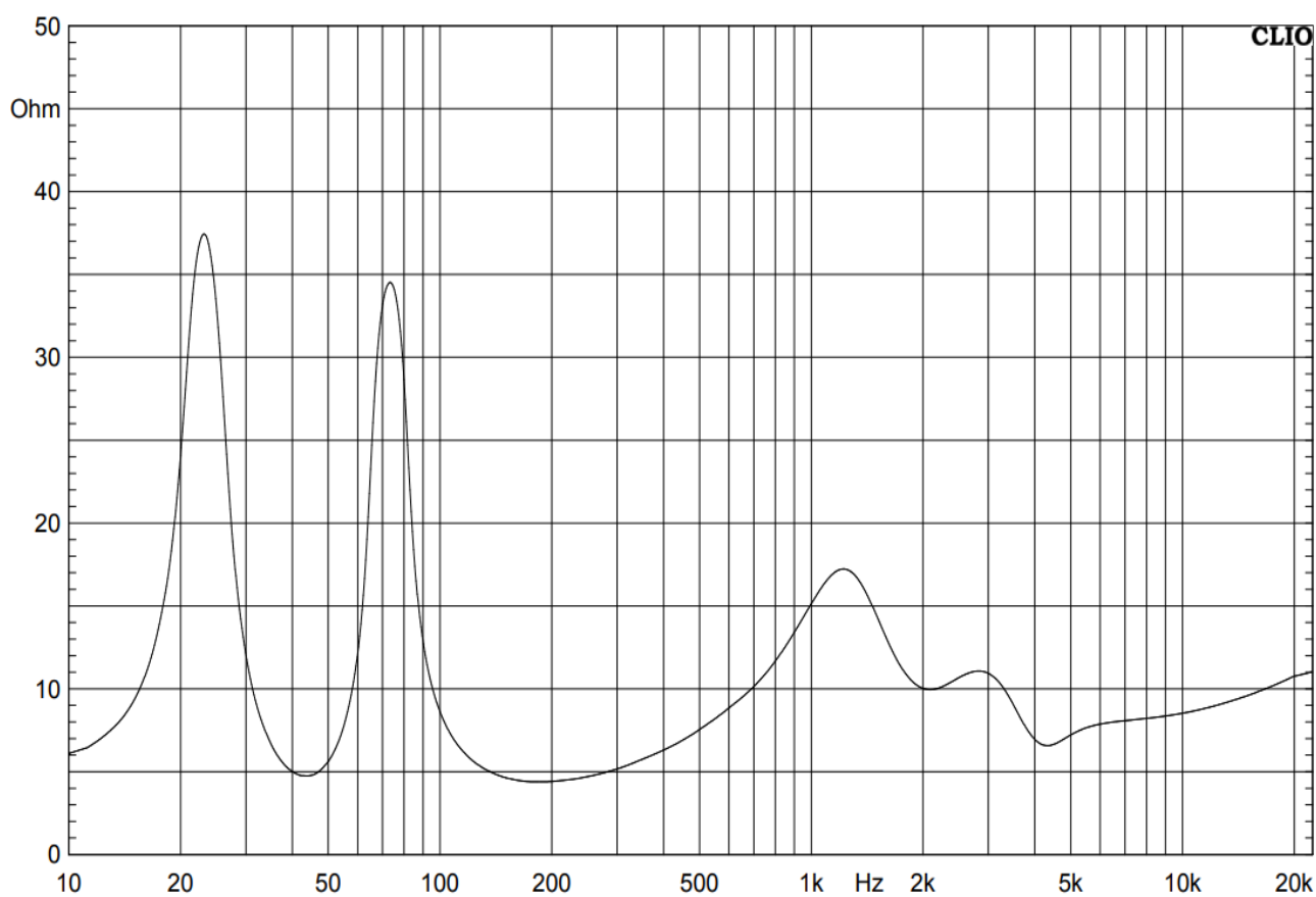
阻抗曲线
