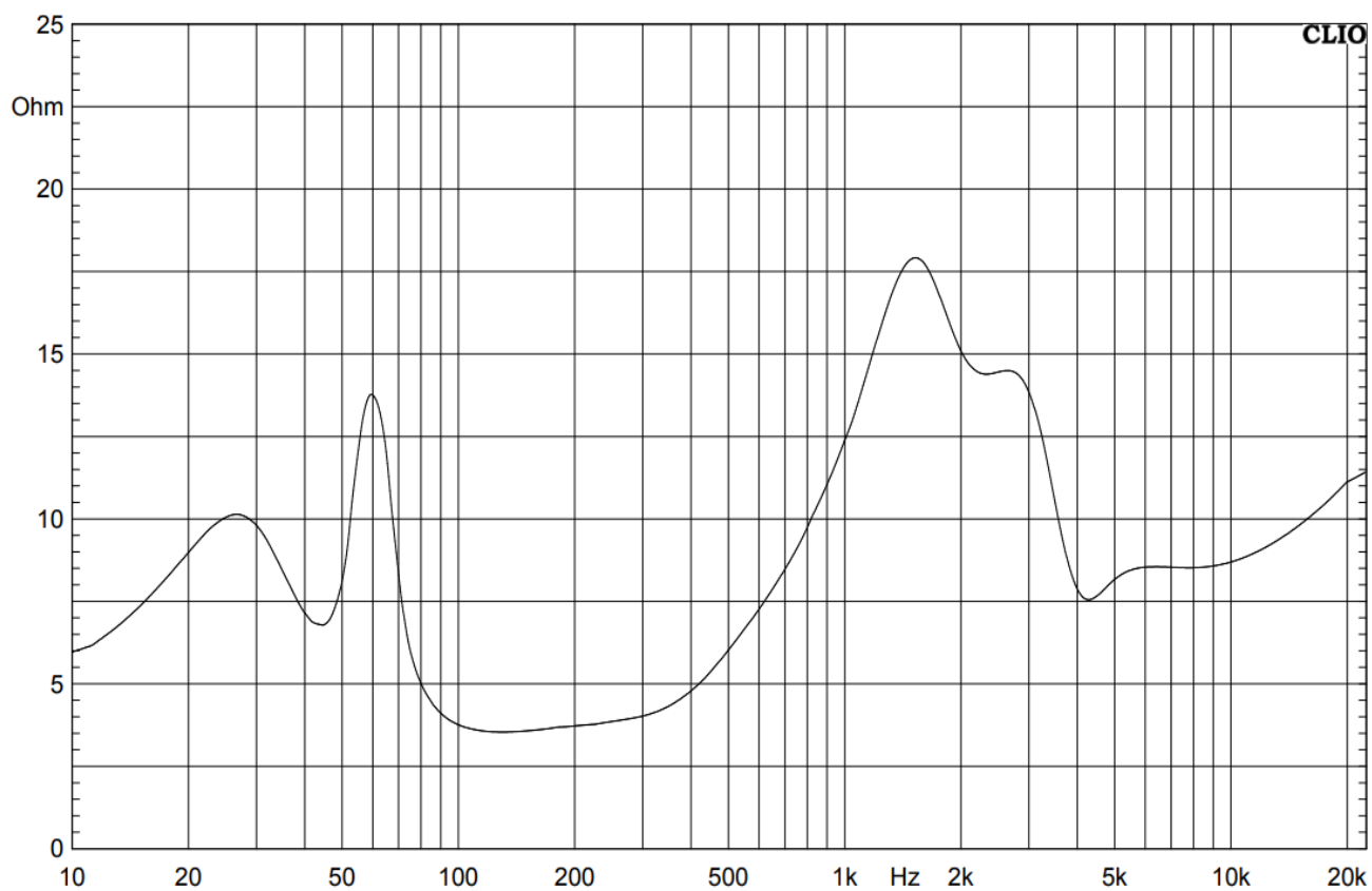
阻抗曲线
