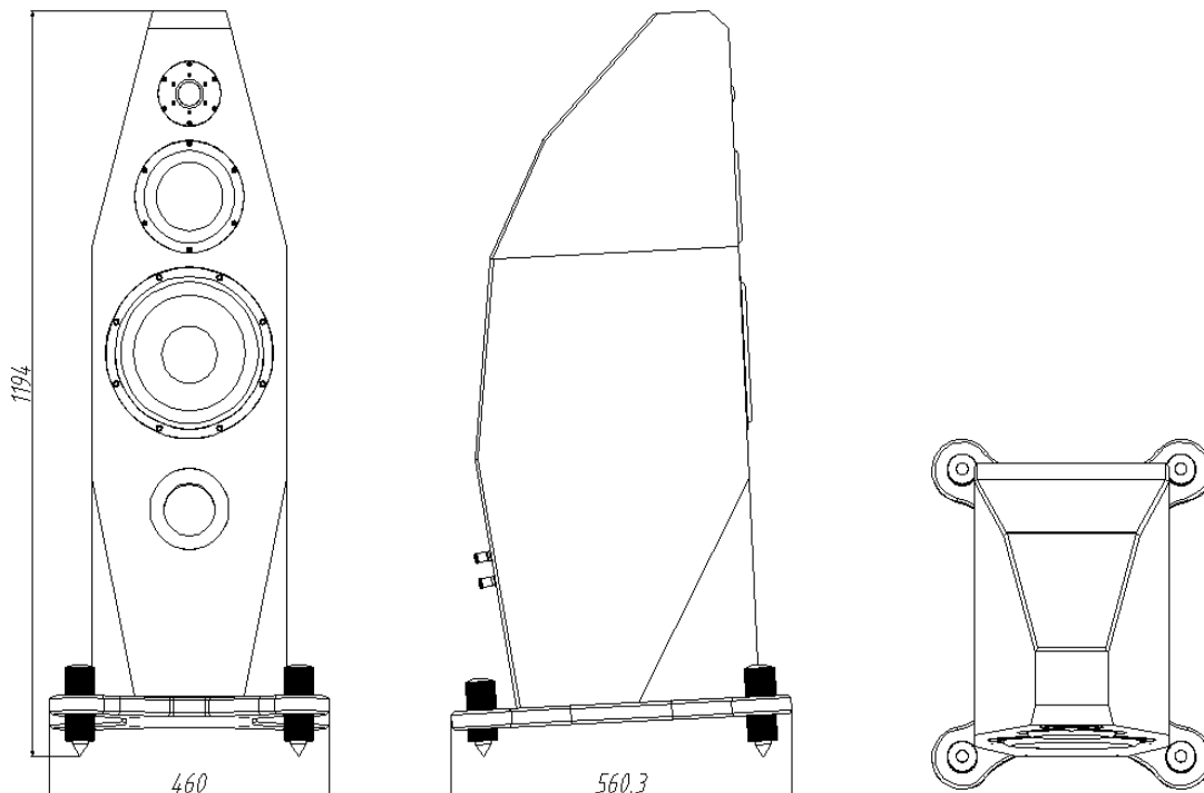
三视图
